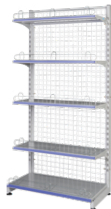
GST03 W900 x D480 x H1820
